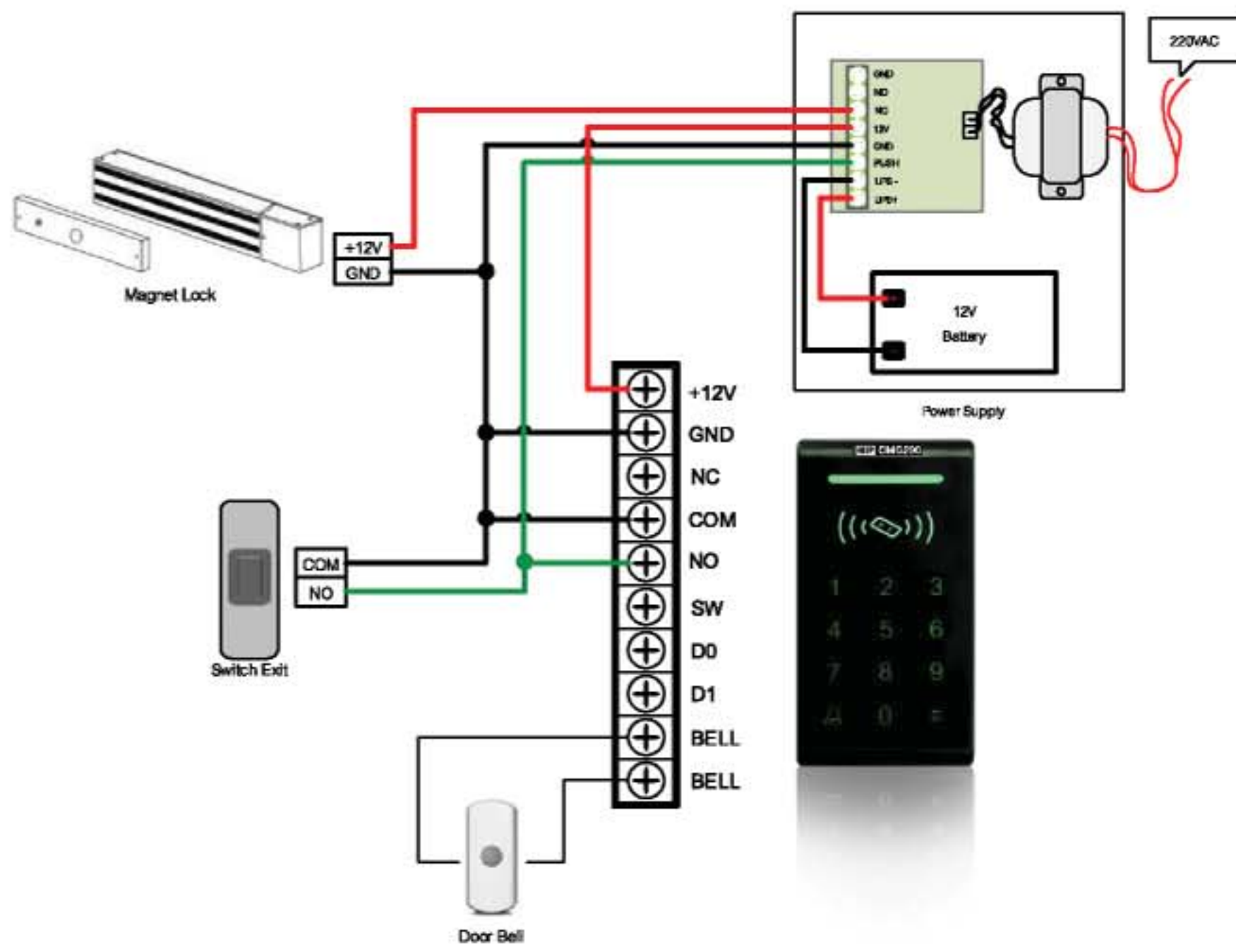
การเชื่อมต่อสำหรับการใช้งาน Standalone ของเครื่อง CMG290
