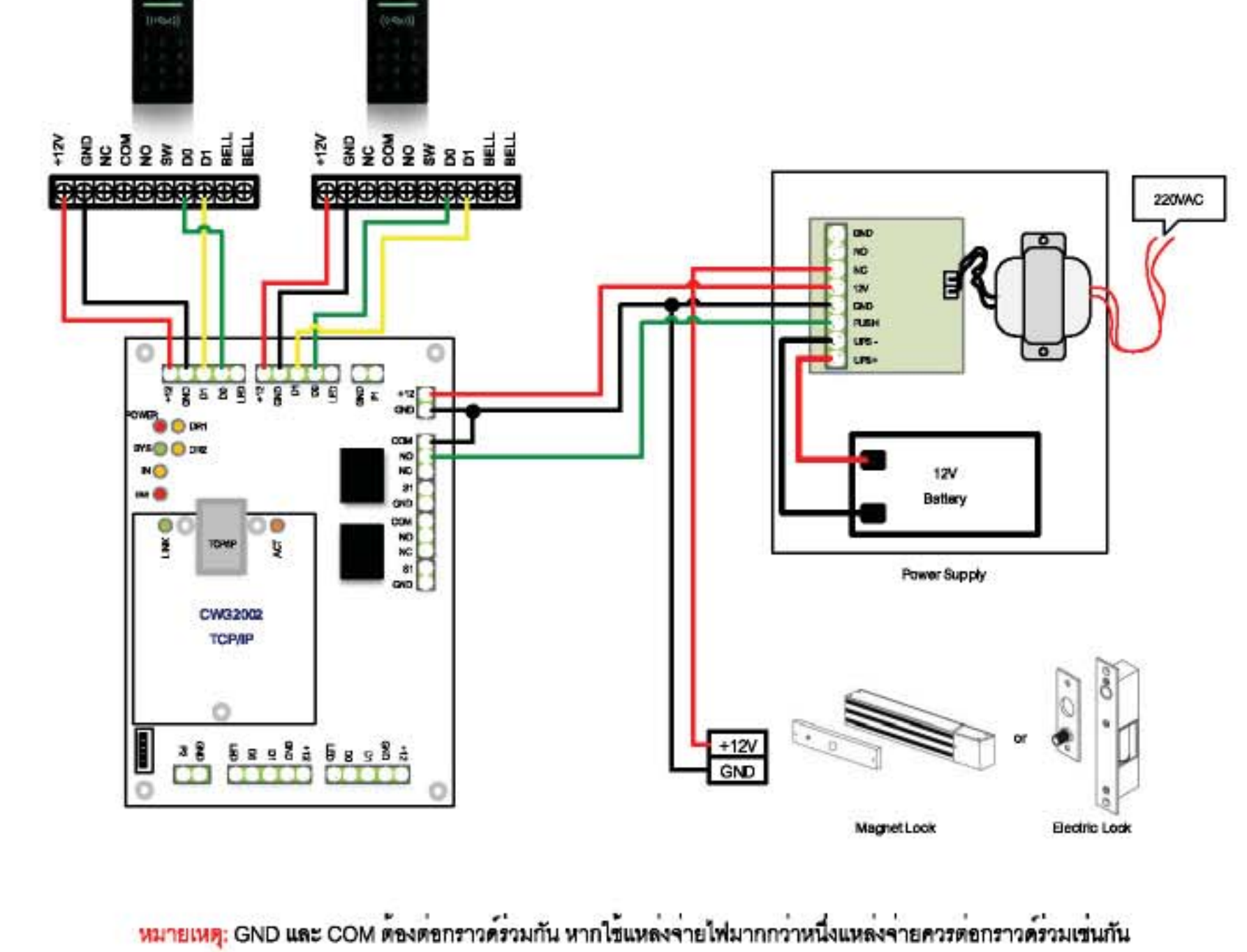
ภาพการเชื่อมต่อเครื่อง CMG290 กับบอร์ด Wiegand
