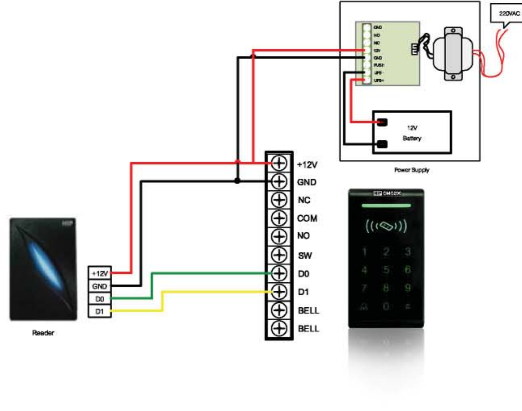
ภาพการเชื่อมต่อขยายเครื่องอ่านบัตรกับเครื่อง CMG290
